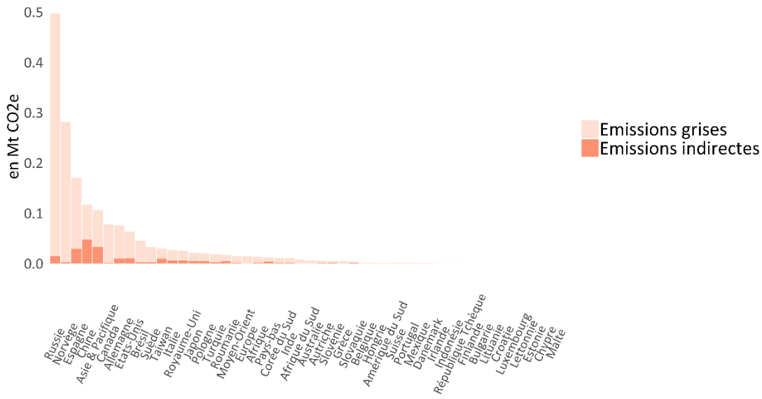
Montant des émissions de PFC par origine géographique
