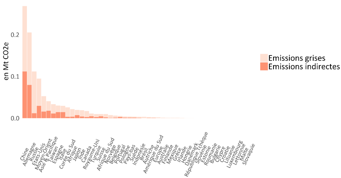
Montant des émissions de SF6 par origine géographique
