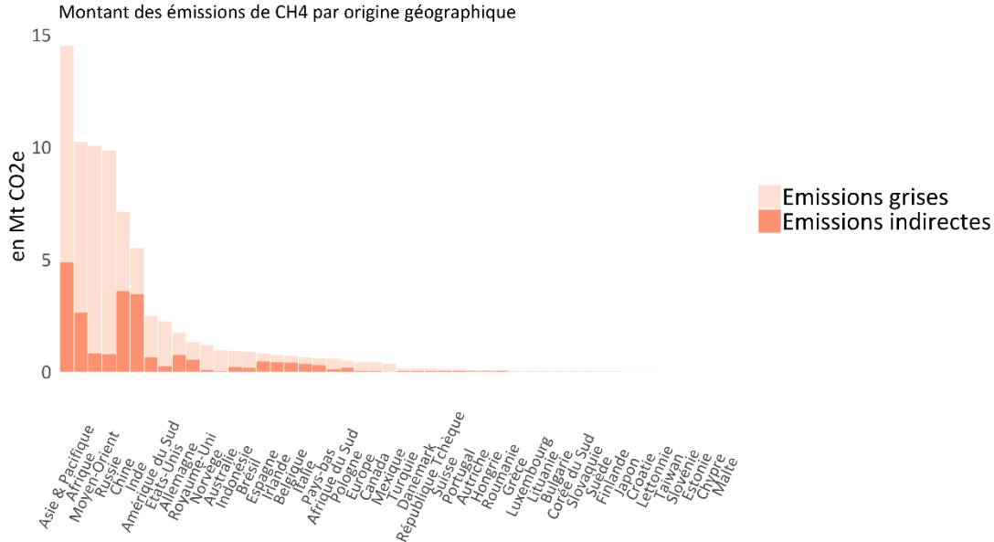
Figure 25: Décomposition des émissions indirectes par zone géographique d'origine
