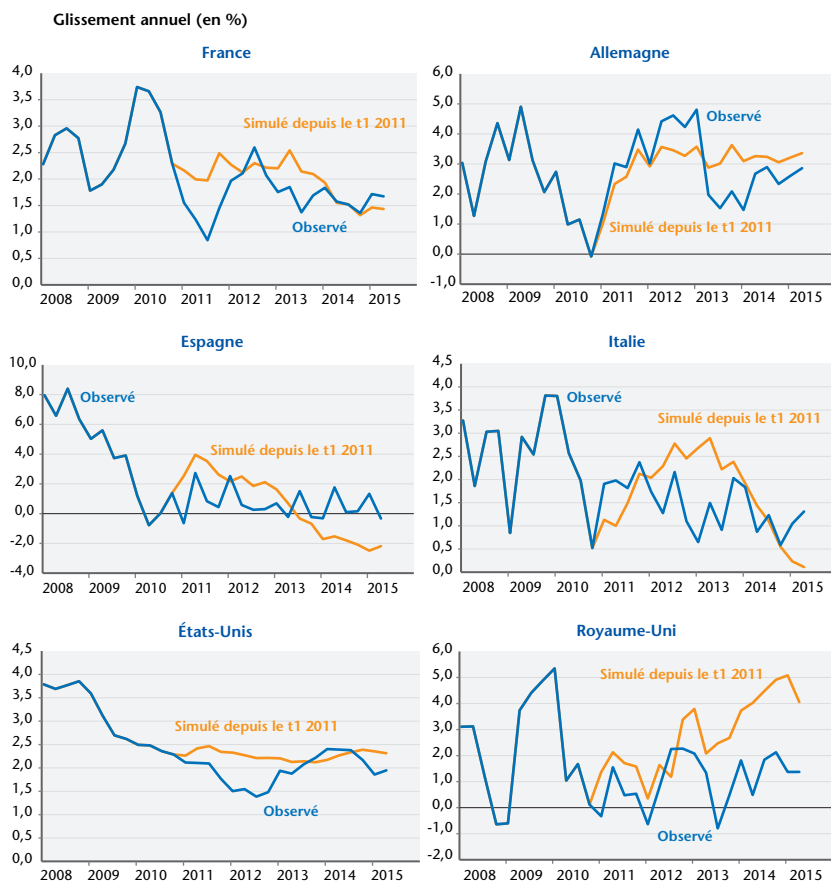
Graphique 6. Simulation dynamique des courbes de Phillips
