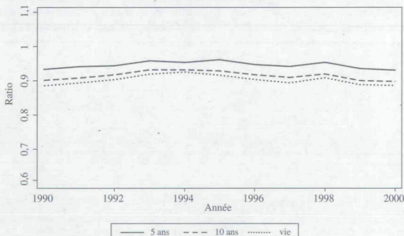
b) Indice d'immobilité
