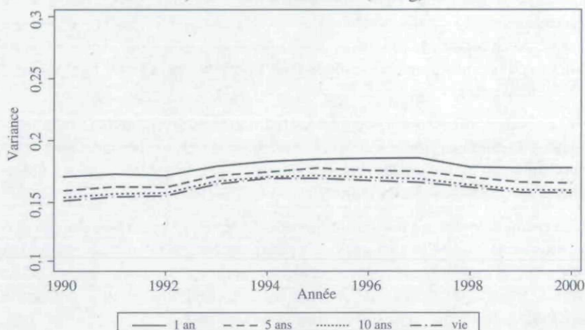
a) Variance des annuités (en log)
