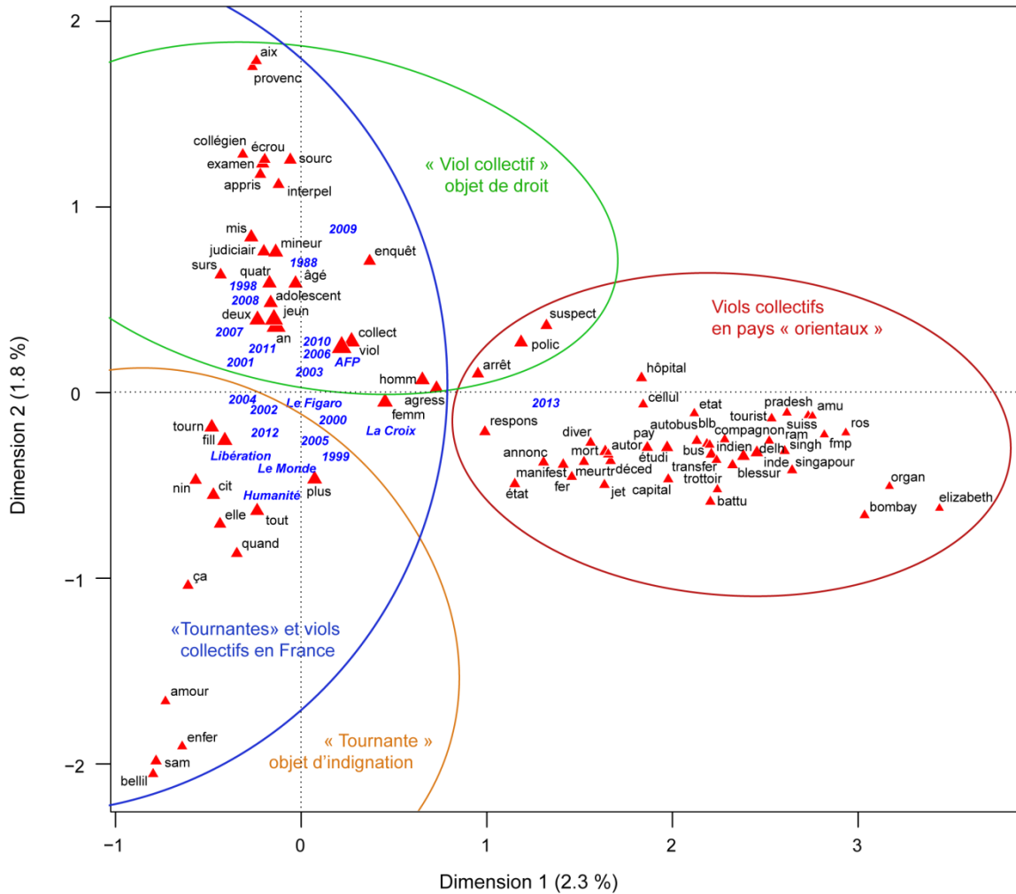
Figure 1 – Analyse des correspondances sur corpus complet.
