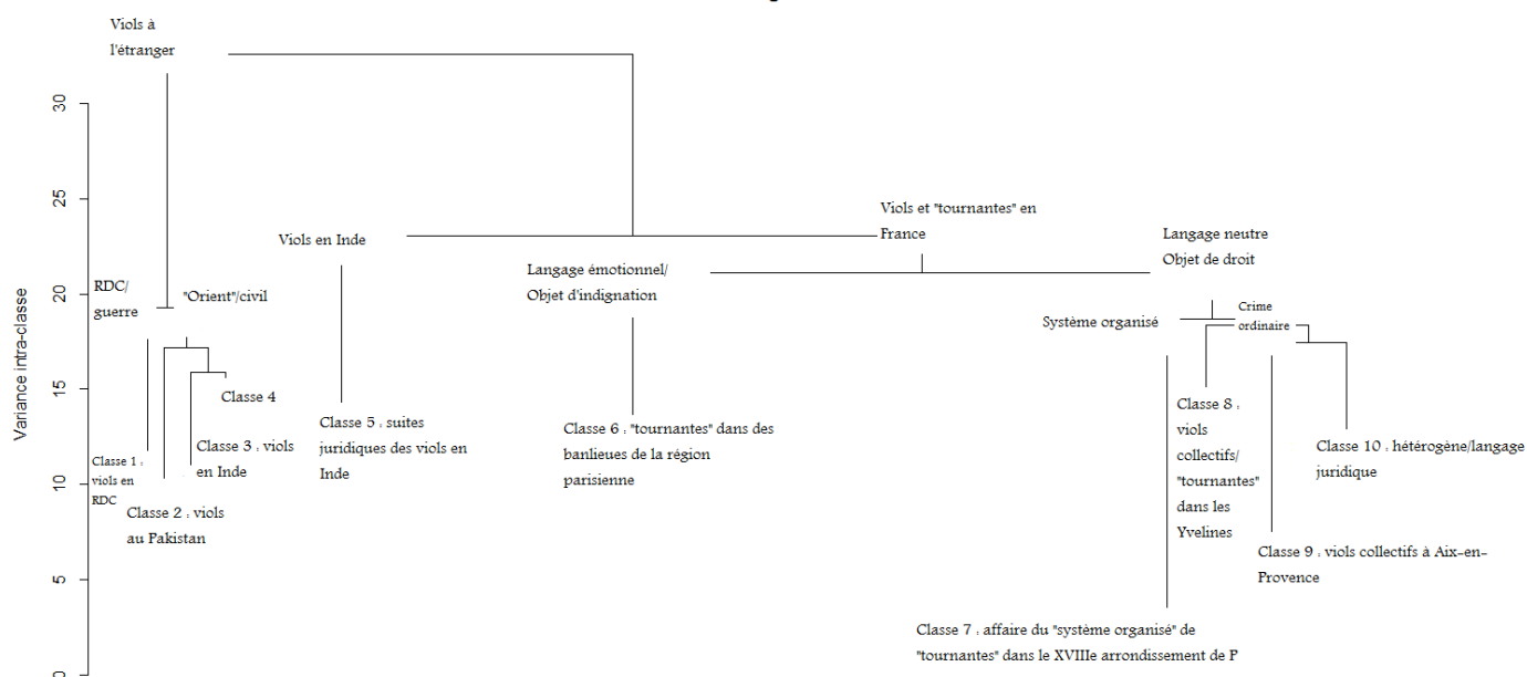
Dendrogramme des documents
