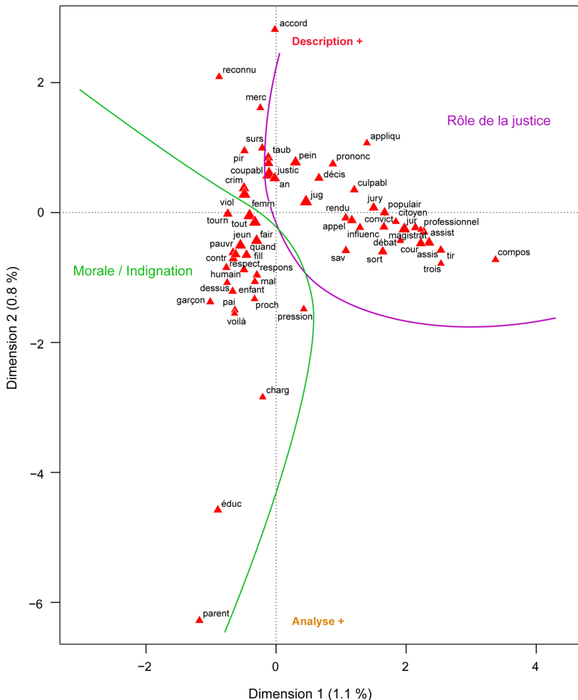
FIGURE 4 – ANALYSE DES CORRESPONDANCES SUR LE CORPUS DE COMMENTAIRES
