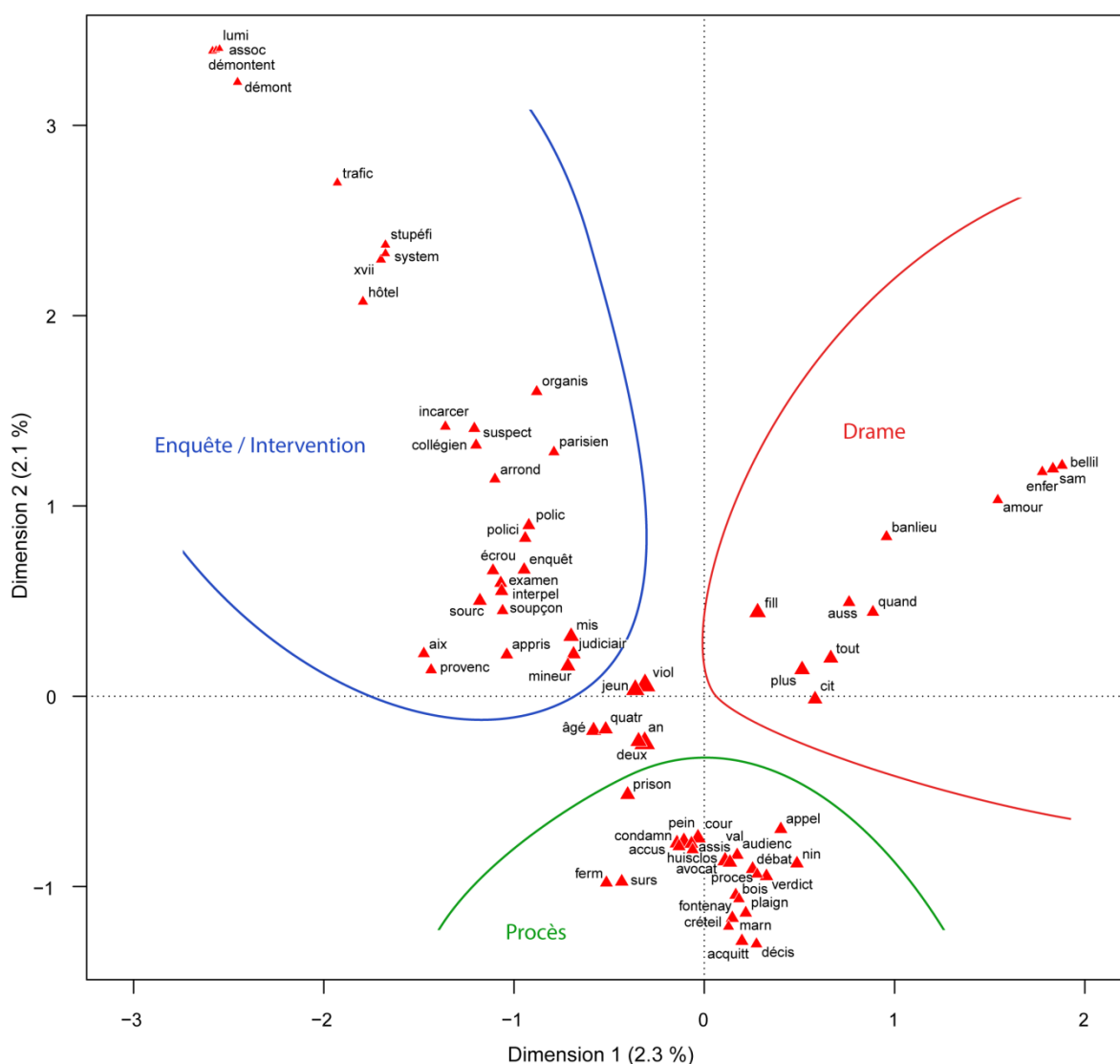
FIGURE 2 – ANALYSE DES CORRESPONDANCES SUR LE SOUS-CORPUS « FRANCE »
