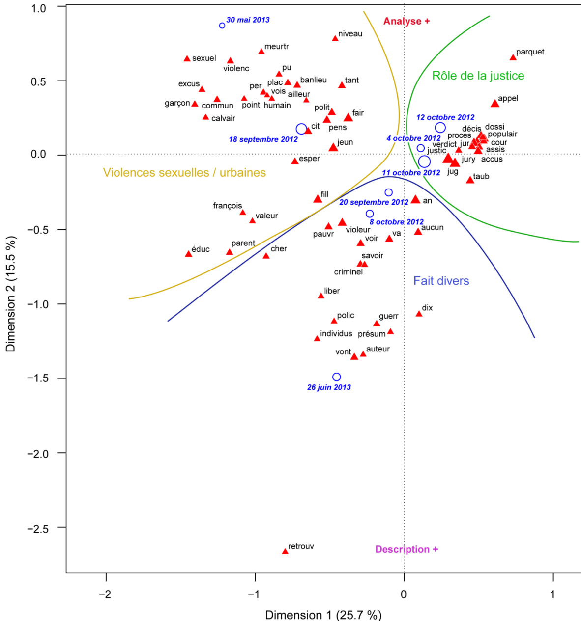
FIGURE 3 – ANALYSE DES CORRESPONDANCES SUR LE CORPUS DE COMMENTAIRES AGREGÉ PAR DATE
