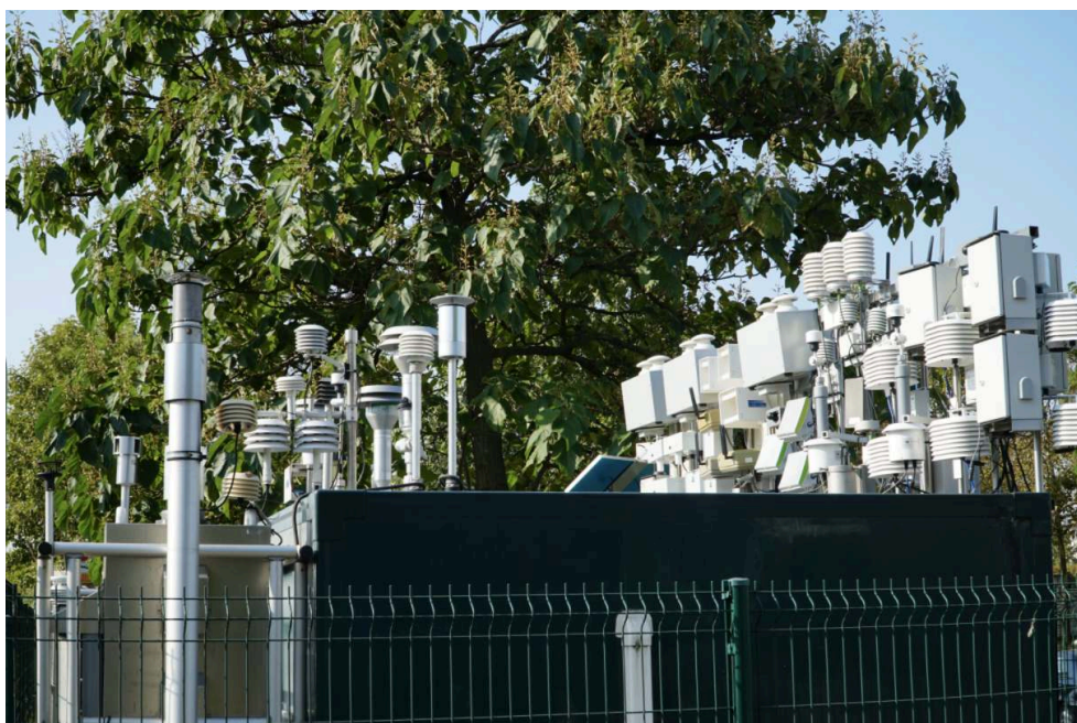
Figure 3 : micro-capteurs du concours installés sur une station de référence pour la mesure de l'air extérieur
