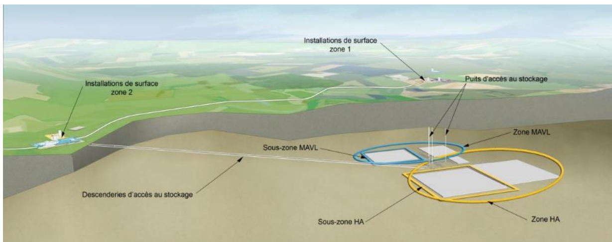
Vue 3D du stockage (scénario de base), (Dossier 2009)
